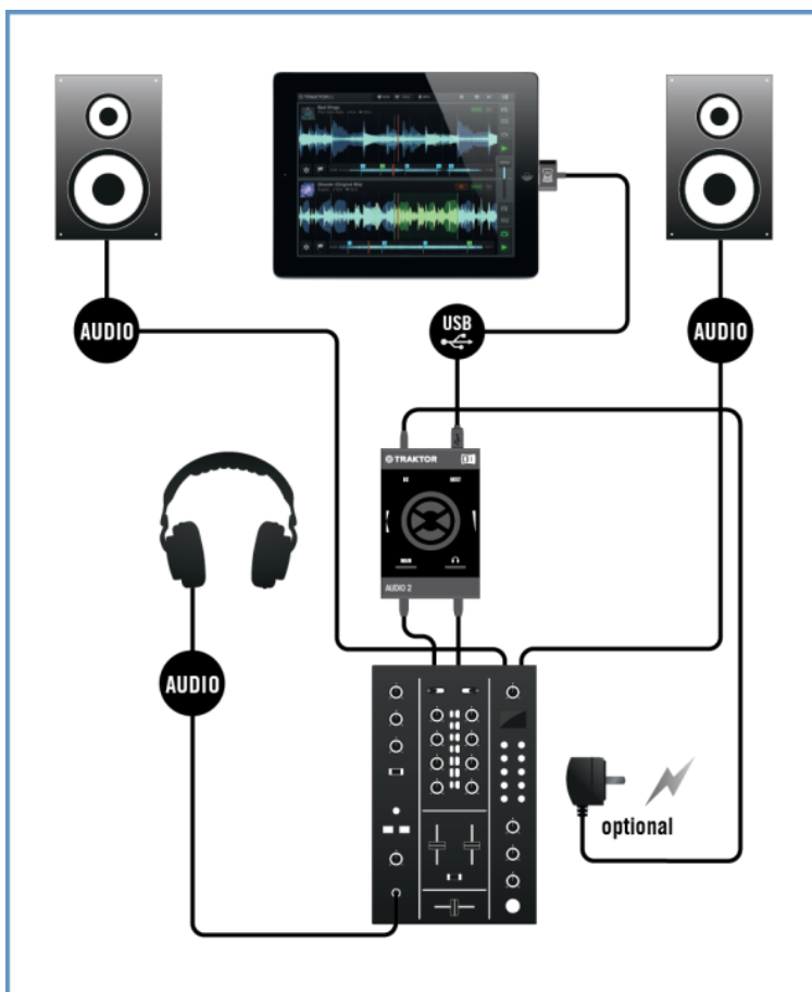
Vue d'ensemble de la configuration de la TA2 avec un appareil iOS utilisé en mode External Mixer.
