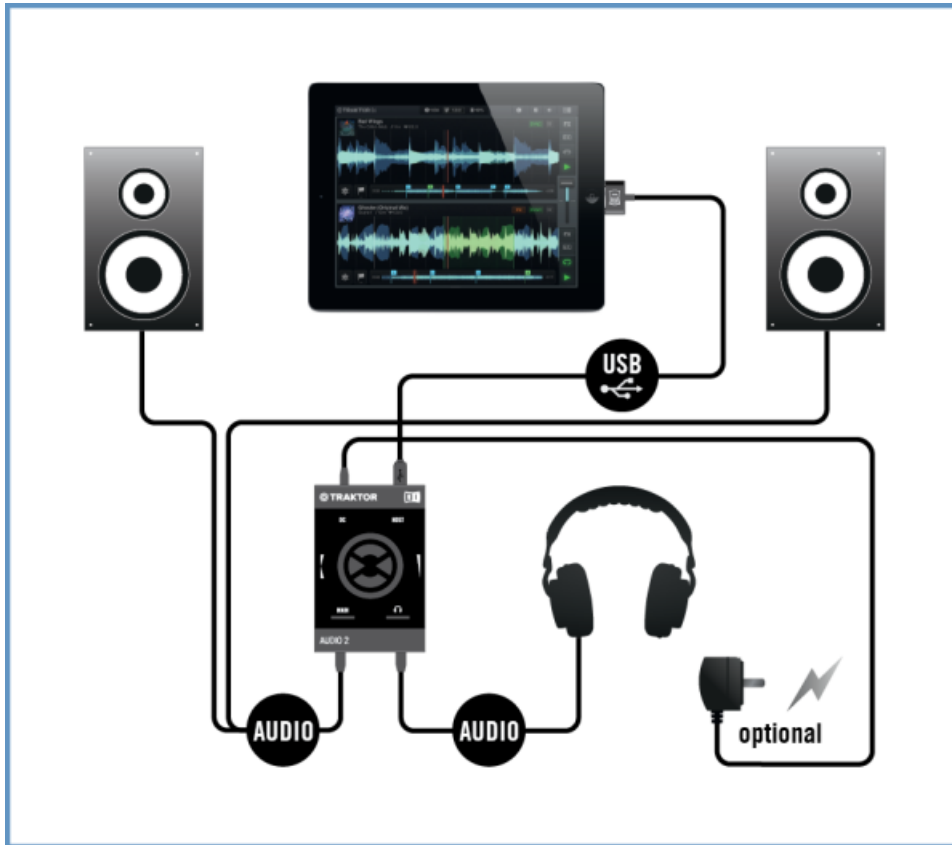
Vue d'ensemble de la configuration de la TA2 avec un appareil iOS utilisé en mode Internal Mixer.
